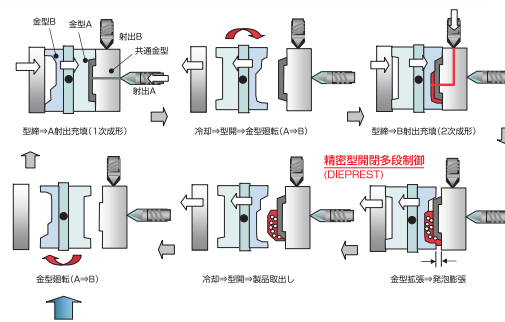
積層射出発泡成形の成形動作フロー
