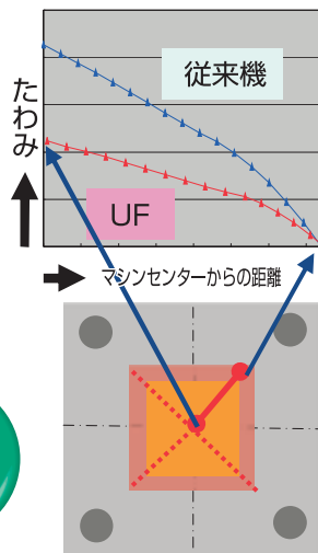
プラテン剛性比較:進化したBOX構造
